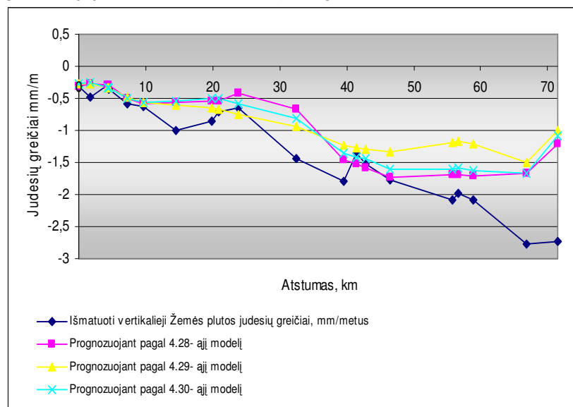
B10 PRIEDAS. Išmatuotų ir prognozuotų vertikalųjų Žemės plutos judesių 5 poligone linijoje Jonava–Gaižiūnai–Palemonas–Kaunas–Kazlų Rūda–Kybartai grafikas
