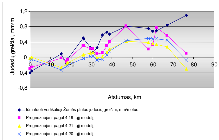
B1 PRIEDAS. Išmatuotų ir prognozuotų vertikalųjų Žemės plutos judesių 1 poligone linijoje Mikytai–Šilutė–Klaipėda–Palanga–Būtingė grafikas
