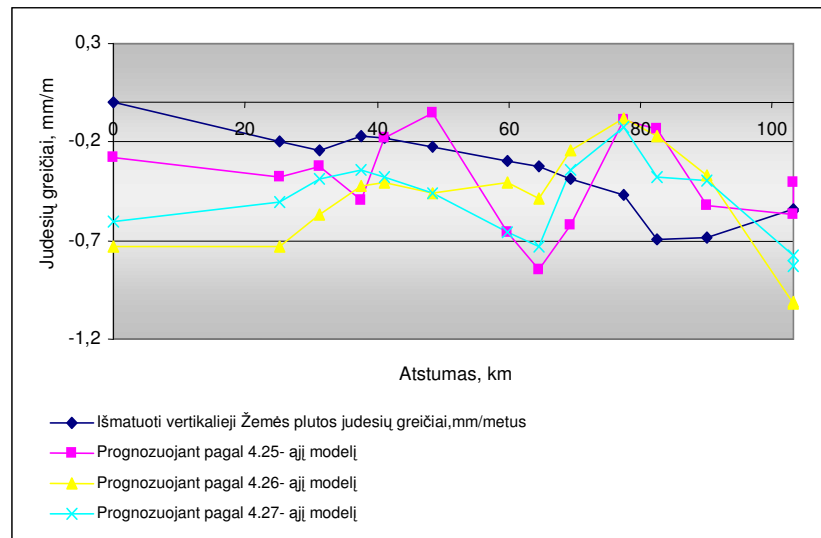
B9 PRIEDAS. Išmatuotų ir prognozuotų vertikalųjų Žemės plutos judesių 3 poligone linijoje Vilnius–Jonava–Jelgava grafikas
