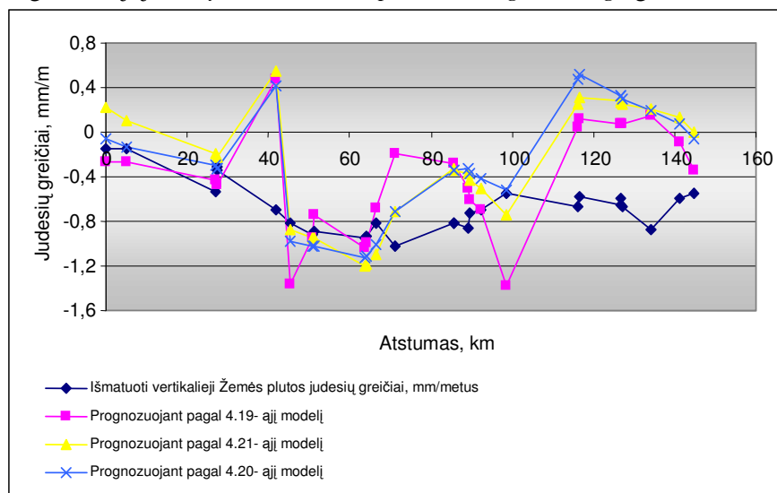
B2 PRIEDAS. Išmatuotų ir prognozuotų vertikalųjų Žemės plutos judesių 1 poligone linijoje Šiauliai–Tauragė–Mikytai grafikas
