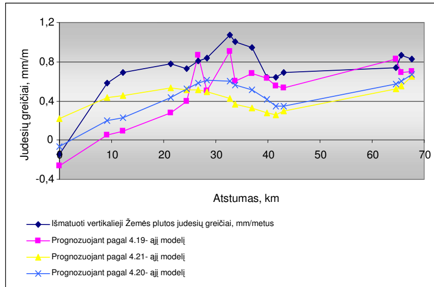
B3 PRIEDAS. Išmatuotų ir prognozuotų vertikalųjų Žemės plutos judesių 1 poligone linijoje Šiauliai–Kuziai–Mažeikiai–Lūšė grafikas
