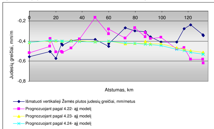
B3 PRIEDAS. Išmatuotų ir prognozuotų vertikalųjų Žemės plutos judesių 1 poligone linijoje Šiauliai–Kuziai–Mažeikiai–Lūšė grafikas
