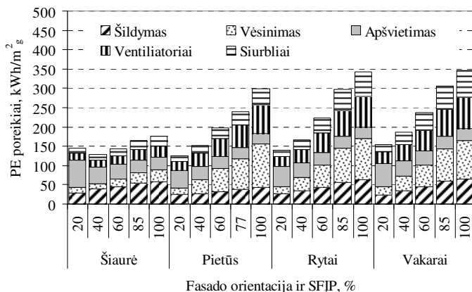
4.28 pav. Stiklo paketo Nr. 4 PE energijos poreikių struktūra
