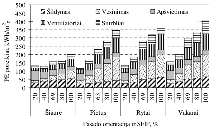
4.29 pav. Stiklo paketo Nr. 5 PE energijos poreikių struktūra
