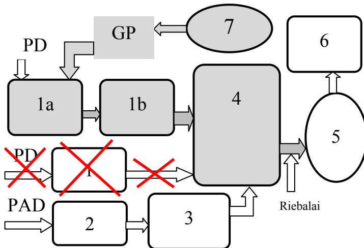
5 pav. Geležies paplavų panaudojimo Utenos valyklos dumblo apdorojimo ūkyje technologinė schema: PD – valykloje susidarantis pirminis dumblas, PAD – valykloje susidarantis perteklinis veiklusis dumblas; GP – geležies paplavyos iš Utenos vandens ruošimo įrenginių; 1 – pirminio dumblo tirštinimas; 1a – pirminio dumblo ir geležies paplavų sumaišymo talpa; 1b – pirminio dumblo ir geležies paplavų tirštinimas; 2 – perteklinio veikiojo dumblo tirštinimas; 3 – perteklinio dumblo apdorojimas utragarsu; 4 – pirminio dumblo su įterptomis paplavomis ir perteklinio dumblo sumaišymas; 5 – dumblo mišinio pūdymas; 6 – pūdyto dumblo sausinimas; 7 – geležies paplavų surinkimo rezervuaras
