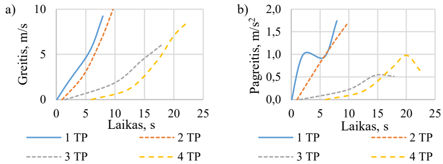
A.8 pav. Keturių pirmųjų TP judėjimo užsidegus žaliai šviesoforo signalui: a) greičio; b) pagreičio priklausomybės nuo laiko 8 šviesoforo ciklo metu
