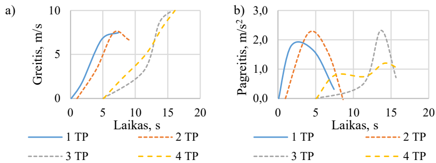
A.1 pav. Keturių pirmųjų TP judėjimo užsidegus žaliajam šviesoforo signalui: a) greičio; b) pagreičio priklausomybės nuo laiko 1 šviesoforo ciklo metu
