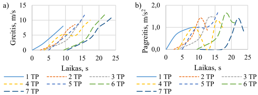
A.9 pav. Septynių pirmųjų TP judėjimo užsidegus žaliai šviesoforo signalui: a) greičio; b) pagreičio priklausomybės nuo laiko 9 šviesoforo ciklo metu
