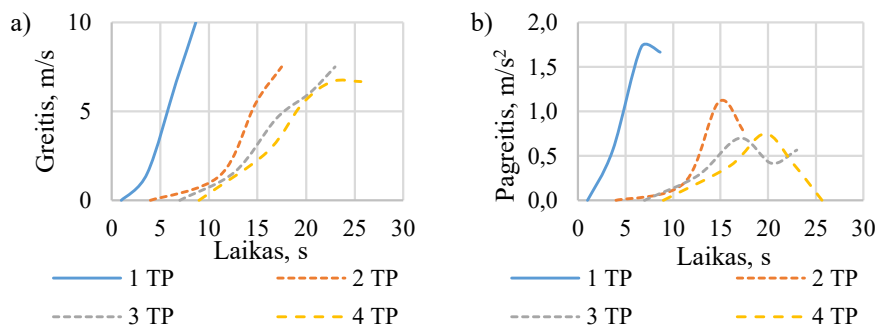
A.6 pav. Keturių pirmųjų TP judėjimo užsidedus žaliajam šviesoforo signalui:
