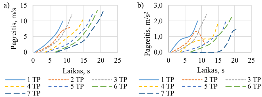
A.10 pav. Septynių pirmųjų TP judėjimo užsidegus žaliajam šviesoforo signalui: a) greičio; b) pagreičio priklausomybės nuo laiko 10 šviesoforo ciklo metu
