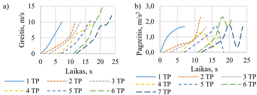
A.3 pav. Septynių pirmųjų TP judėjimo užsidegus žaliajam šviesoforo signalui: a) greičio; b) pagreičio priklausomybės nuo laiko 3 šviesoforo ciklo metu
