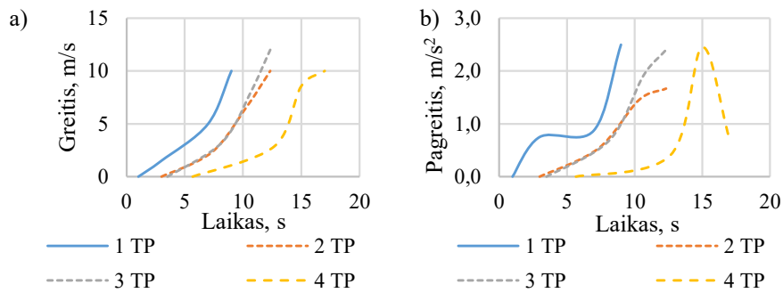
A.2 pav. Keturių pirmųjų TP judėjimo užsidegus žaliajam šviesoforo signalui: a) greičio; b) pagreičio priklausomybės nuo laiko 2 šviesoforo ciklo metu
