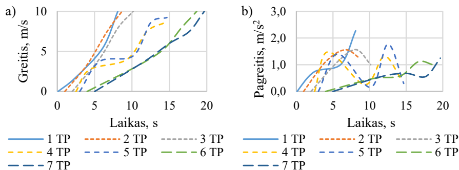
A.4 pav. Septynių pirmųjų TP judėjimo užsidedus žaliajam šviesoforo signalui:
