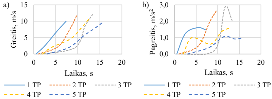
A.7 pav. Penkių pirmųjų TP judėjimo užsidegus žaliai šviesoforo signalui: a) greičio; b) pagreičio priklausomybės nuo laiko 7 šviesoforo ciklo metu
