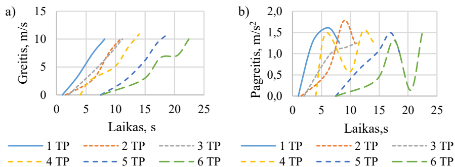
A.5 pav. Šešių pirmųjų TP judėjimo užsidedus žaliajam šviesoforo signalui:
