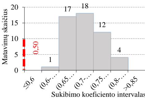
E.9 pav. Skaitinės charakteristikos sukibimo koeficiento AC 11 VS dangos D(IV) užpildo kelio Nr. A4 ruožo
