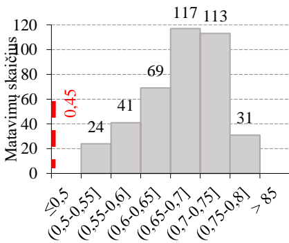
E.2 pav. Skaitinės charakteristikos sukibimo koeficiento paviršiaus aparado dangos D_{(IV)} užpildo kelio Nr. 3404, matavimo 2
