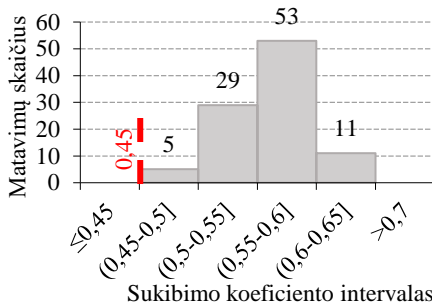
E.1 pav. Skaitinės charakteristikos sukibimo koeficiento paviršiaus aparado dangos D_{(IV)} užpildo kelio Nr. 3404, matavimo 1
