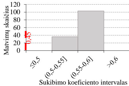
E.1 pav. Skaitinės charakteristikos sukibimo koeficiento paviršiaus aparado dangos D_{(IV)} užpildo kelio Nr. 3404, matavimo 1
