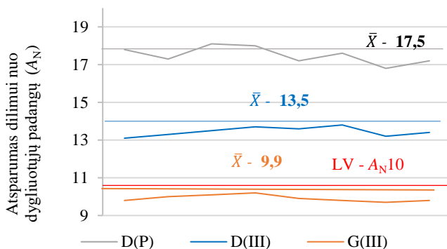
F.4 pav. Atsparumas dilimui nuo dygliuotųjų padangų ( A_N ). Fig. F.4. Abrasion from studded tyres ( A_N )
