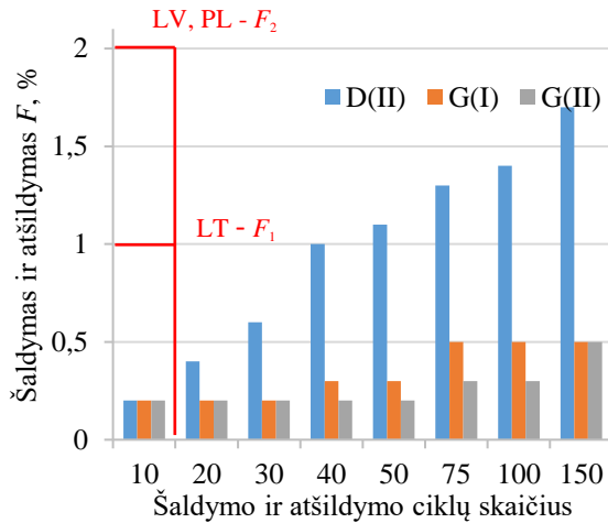
F.7 pav. Atsparumas šaldymui ir atšildymui Fig. F.7. Resistance to freezing and thawing
