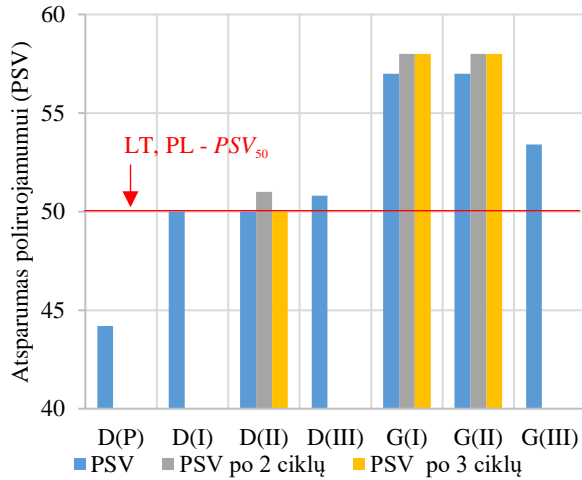
F.6 pav. Atsparumas poliruojamumui (PSV) Fig. F.6. Impact resistance (PSV)
