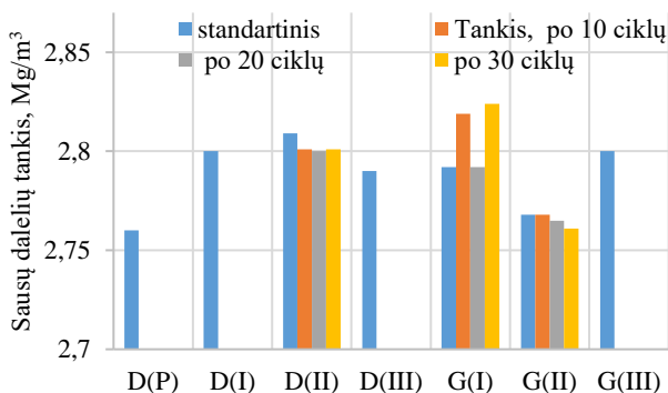
F.5 pav. Sausų dalelių tankio tyrimų rezultatai Fig. F.5. Determination results of particle density
