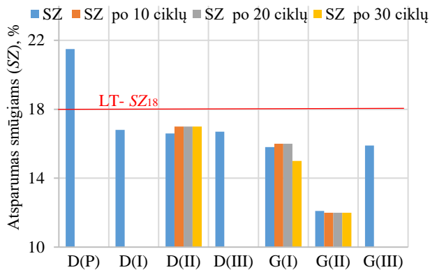
F.3 pav. Atsparumas smūgiams (SZ) Fig. F.3. Impact value (SZ)
