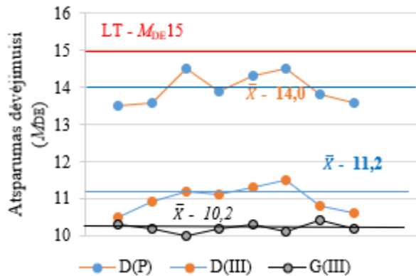
F.1 pav. Atsparumas dėvėjimuisi (mikro Devalio koeficientas) ( M_{DE} ) Fig. F.1. Resistance to wear (micro-Deval) ( M_{DE} )
