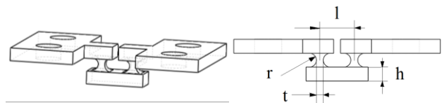
Fig. 6 Tilting flexure hinge
