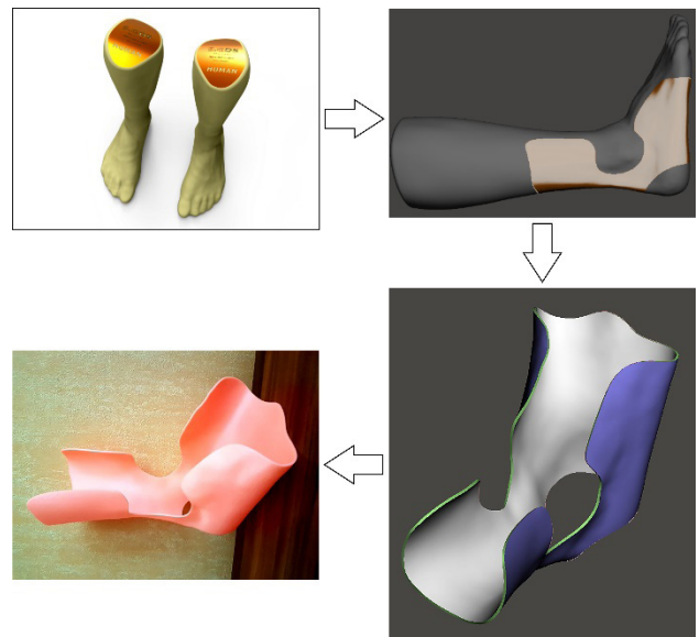
4 paveikslas. Ortopedinio įtvaro 3D modeliavimo ir gamybos procesas
