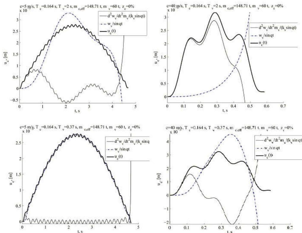
1.9 pav. Tiltų įlinkio u_c kaita, važiuojant transporto priemonei skirtingais greičiais c , esant skirtingiems pakabos savųjų svyravimų dažniams f_v .
